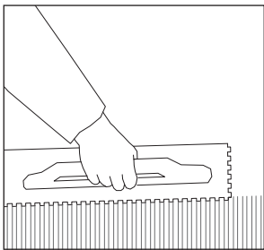
Abb. 4 Floating-Buttering-Verfahren: Vollflächiges Auftragen des mineralischen Klebemörtels mit einer Zahnraufel auf den Untergrund im Bereich des Brandriegels.
