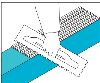
Abb. 5 Auch auf der Rückseite des Brandriegels ist der mineralische Klebermörtel mit einer Zahnraufel vollflächig in der Gegenrichtung zum Kleber- auftrag auf den Untergrund aufzutragen.
