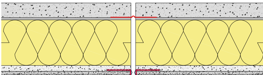
Detailzeichnung D_099
