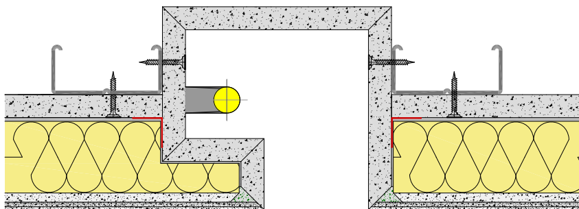
Detailzeichnung D_ 076
