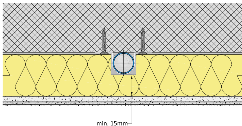
Detailzeichnung D_078
