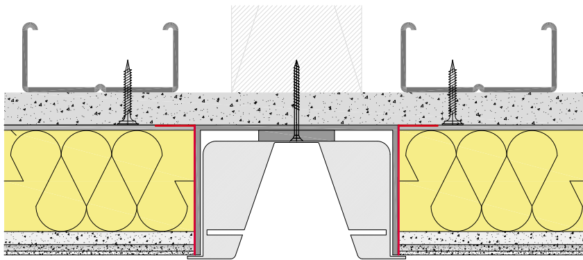
Detailzeichnung D_057
