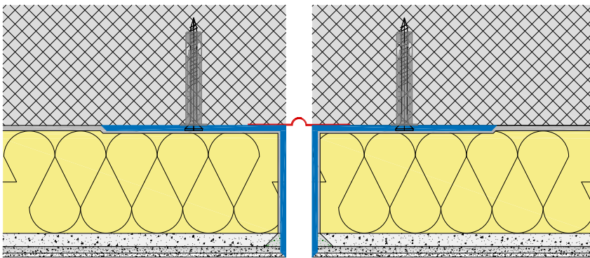
Detailzeichnung D_053
