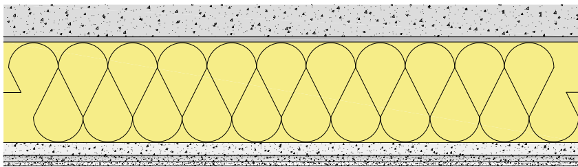
Detailzeichnung D_002
